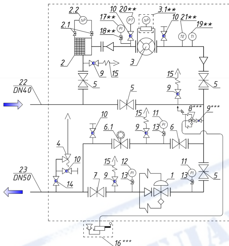
ВИД А
